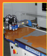
Doppia postazione di lavoro (solo su versioni "888") Double working area (only for "888" models)
